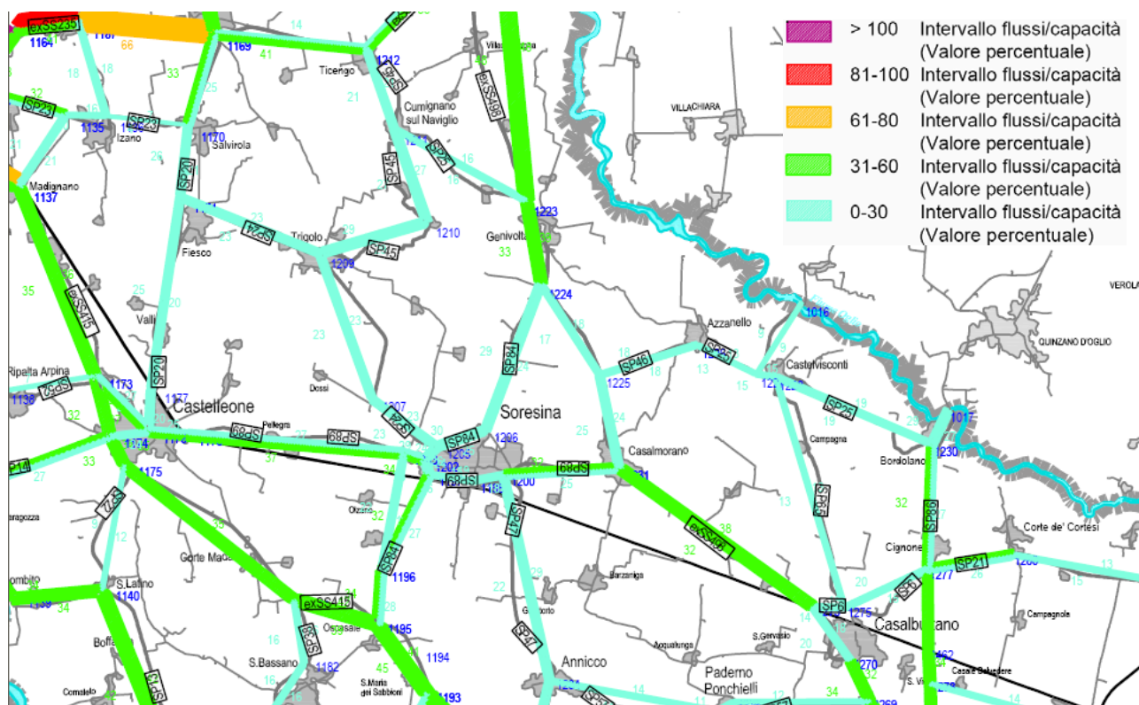
Figura 3-8 Flussi di traffico/capacità della rete viaria principale dell'ambito della Media Pianura Cremonese (Note: flusso ore 8.00-9.00 - veicoli omogeneizzati)
